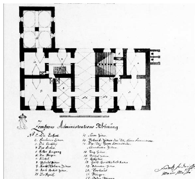
План приземља и спрата Грашалковићеве палате из 1887. год.
