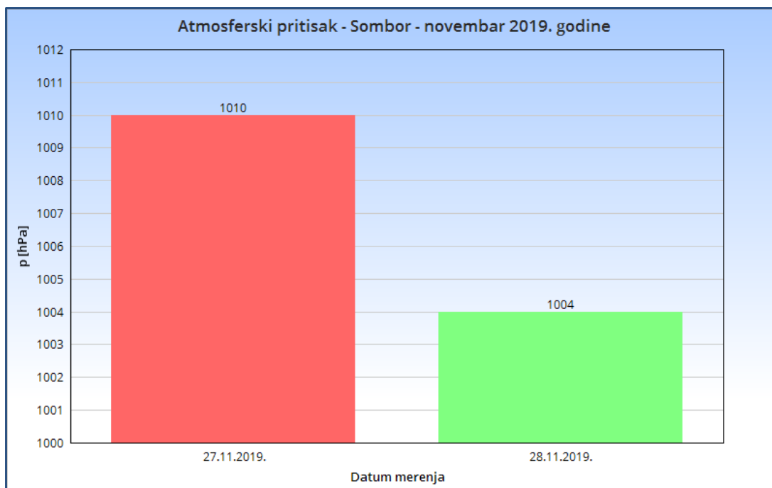
Slika 2.3. Atmosferski pritisak - Sombor novembar 2019. godine
