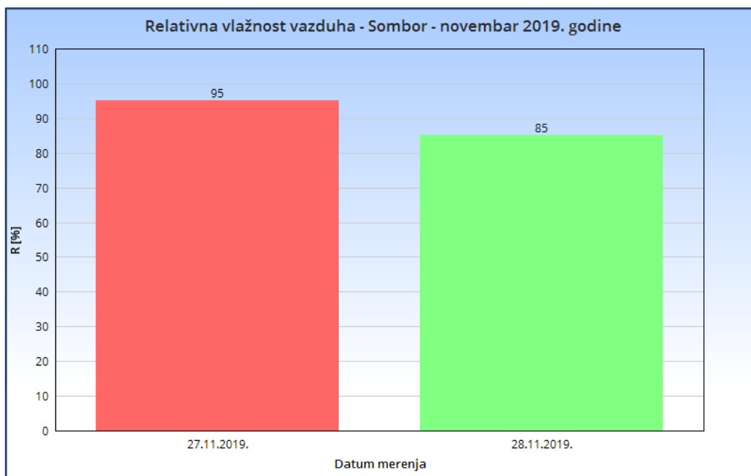
Slika 2.2. Relativna vlažnost vazduha - Sombor novembar 2019. godine
