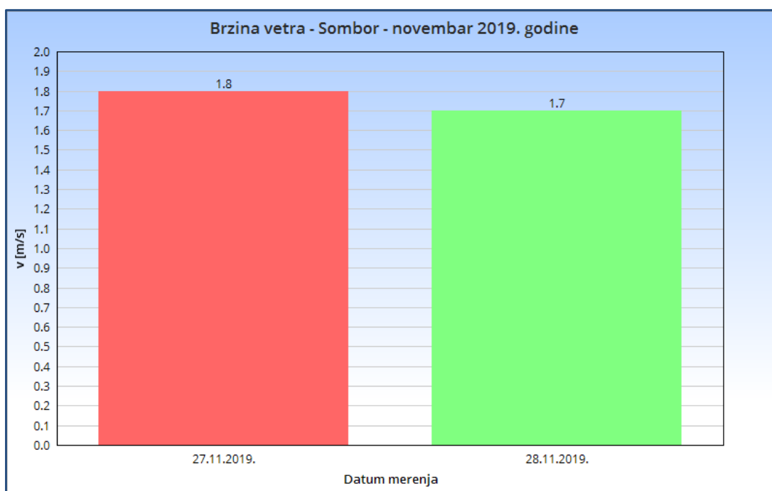
Slika 2.4. Brzina vetra - Sombor novembar 2019. godine
