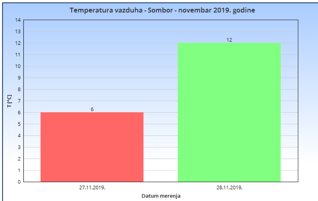
Slika 2.1. Temperatura vazduha - Sombor novembar 2019. godine
