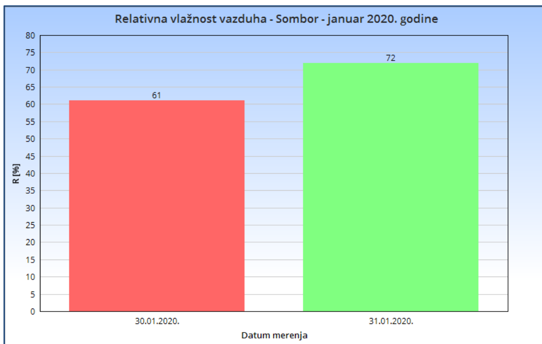
Slika 2.2. Relativna vlažnost vazduha - Sombor januar 2020. godine
