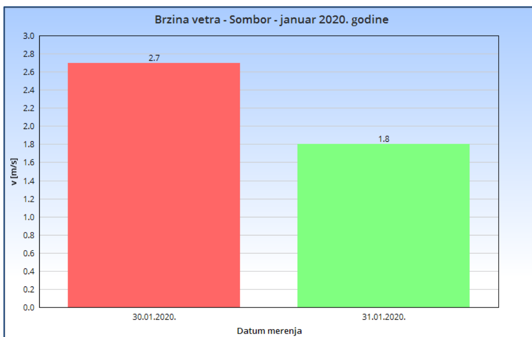
Slika 2.4. Brzina vetra - Sombor januar 2020. godine
