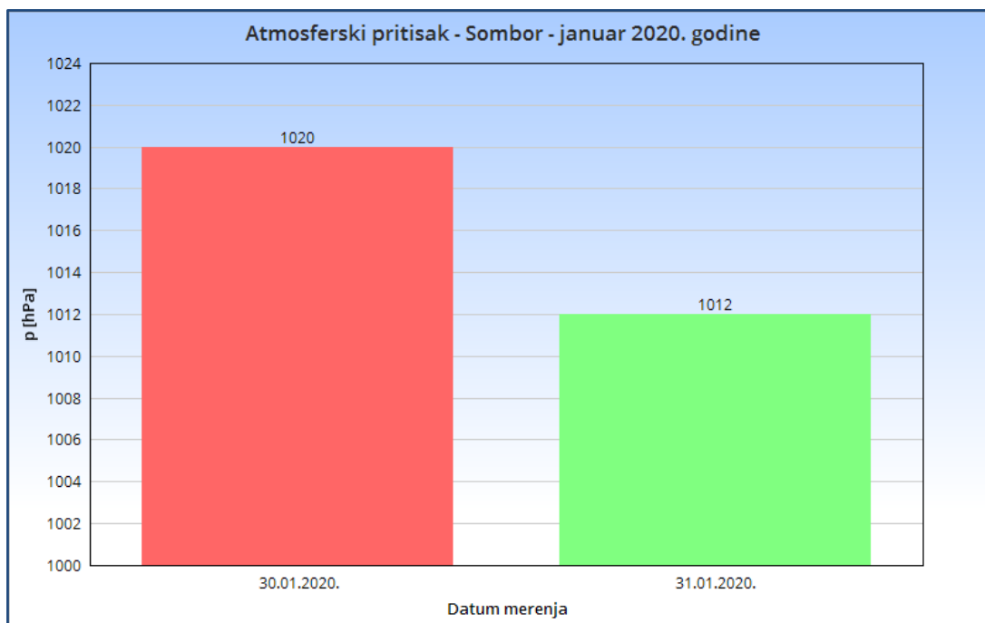
Slika 2.3. Atmosferski pritisak - Sombor januar 2020. godine
