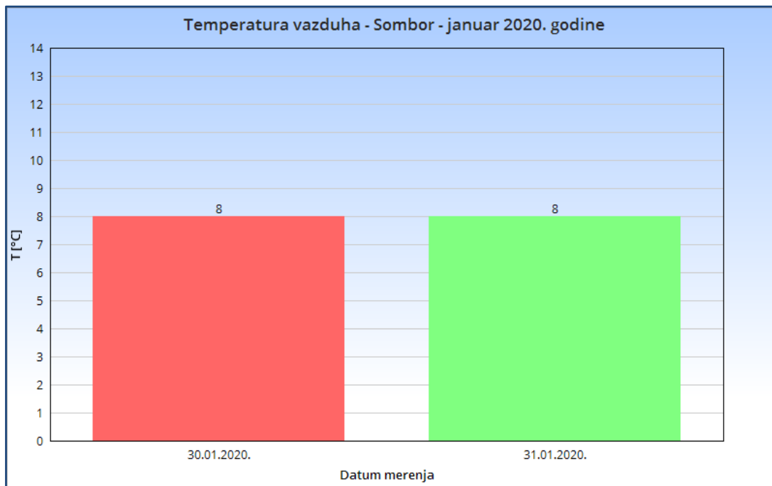
Slika 2.1. Temperatura vazduha - Sombor januar 2020. godine
