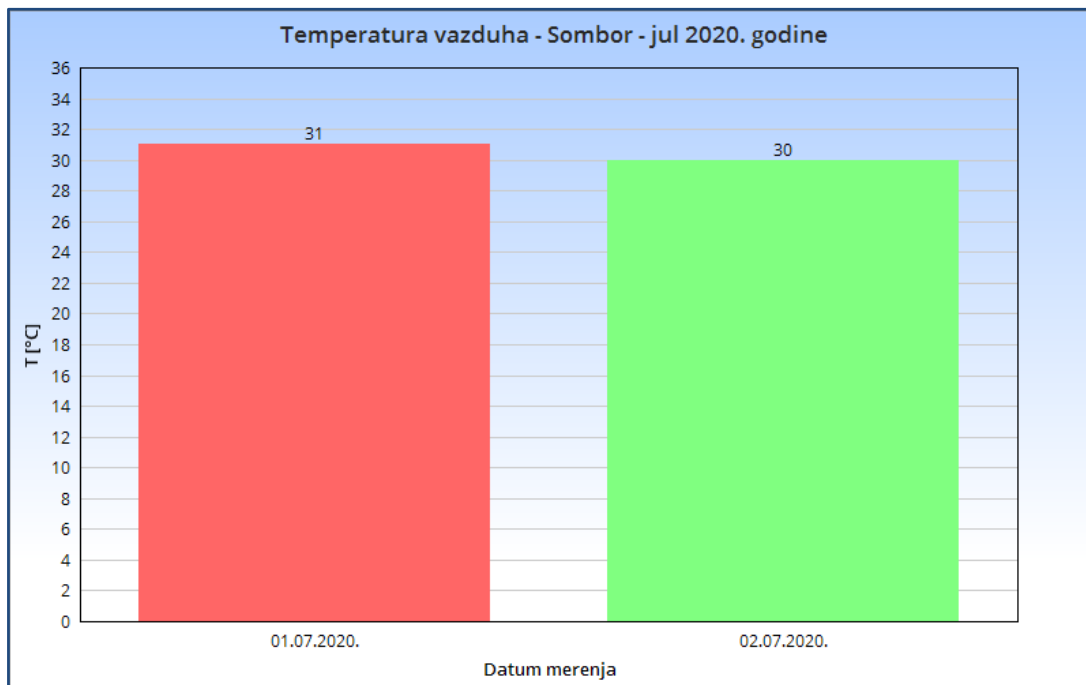
Slika 2.1. Temperatura vazduha - Sombor jul 2020. godine
