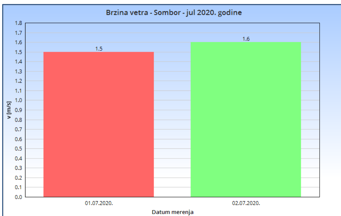
Slika 2.4. Brzina vetra - Sombor jul 2020. godine
