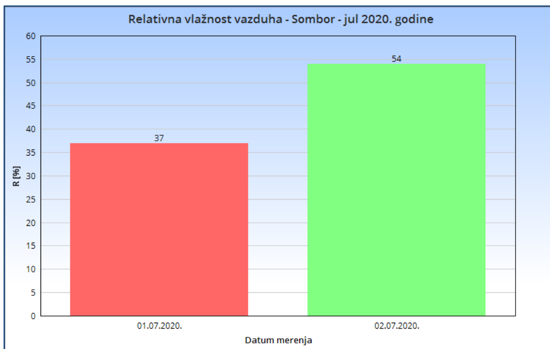
Slika 2.2. Relativna vlažnost vazduha - Sombor jul 2020. godine
