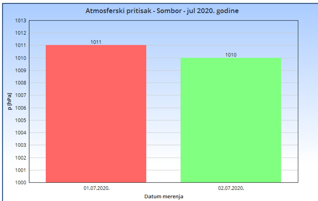
Slika 2.3. Atmosferski pritisak - Sombor jul 2020. godine
