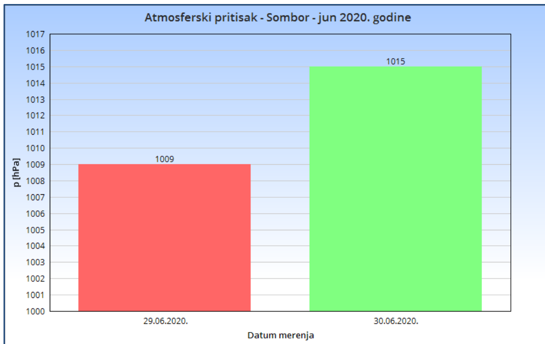
Slika 2.3. Atmosferski pritisak - Sombor jun 2020. godine
