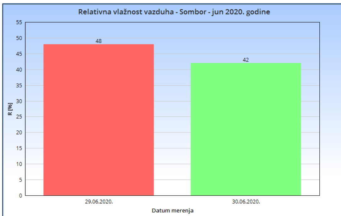
Slika 2.2. Relativna vlažnost vazduha - Sombor jun 2020. godine
