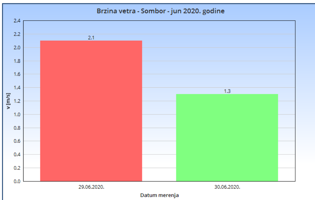
Slika 2.4. Brzina vetra - Sombor jun 2020. godine
