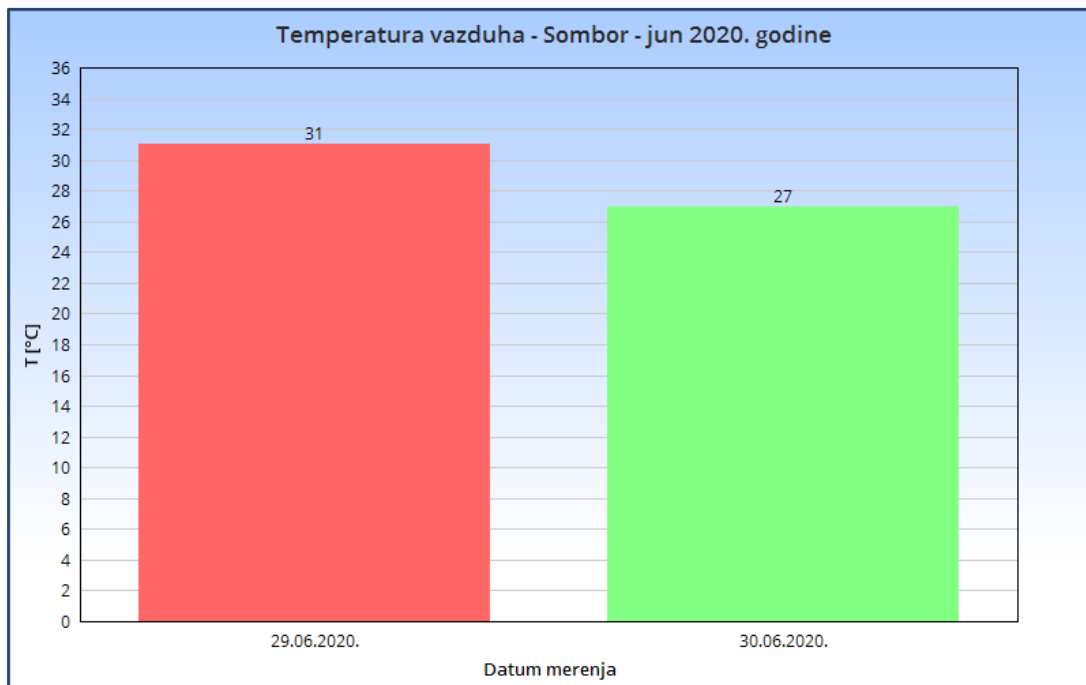
Slika 2.1. Temperatura vazduha - Sombor jun 2020. godine
