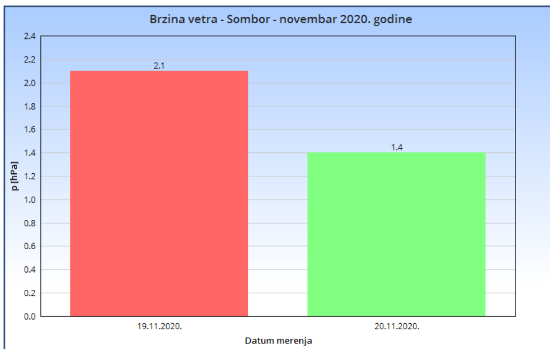
Slika 2.4. Brzina vetra - Sombor novembar 2020. godine
