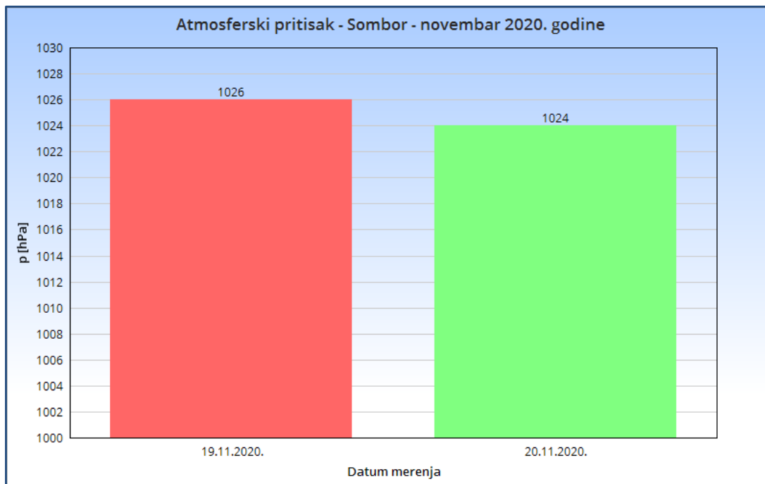
Slika 2.3. Atmosferski pritisak - Sombor novembar 2020. godine
