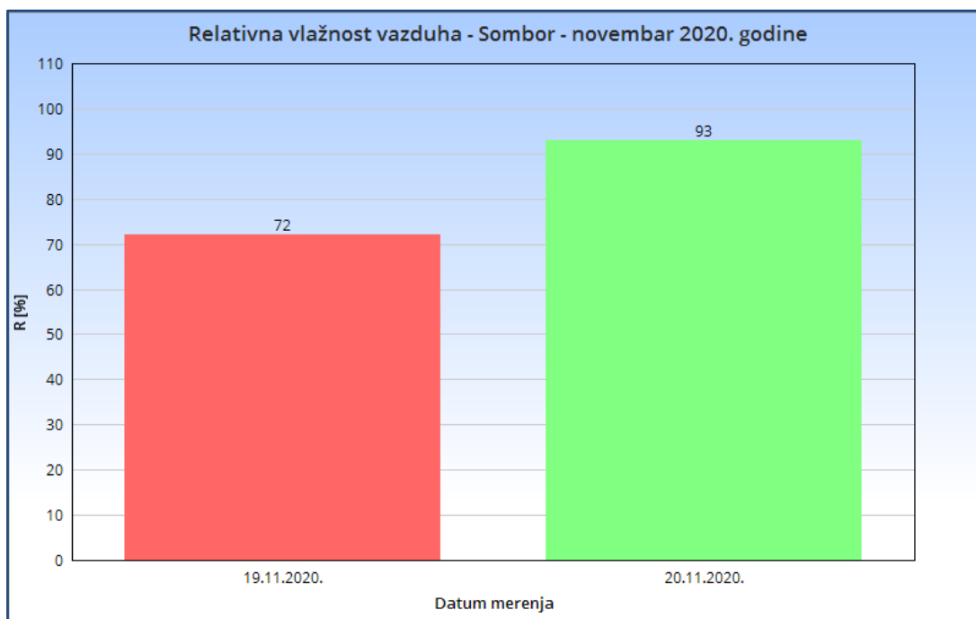
Slika 2.2. Relativna vlažnost vazduha - Sombor novembar 2020. godine
