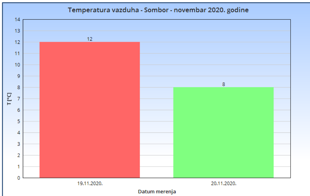
Slika 2.1. Temperatura vazduha - Sombor novembar 2020. godine
