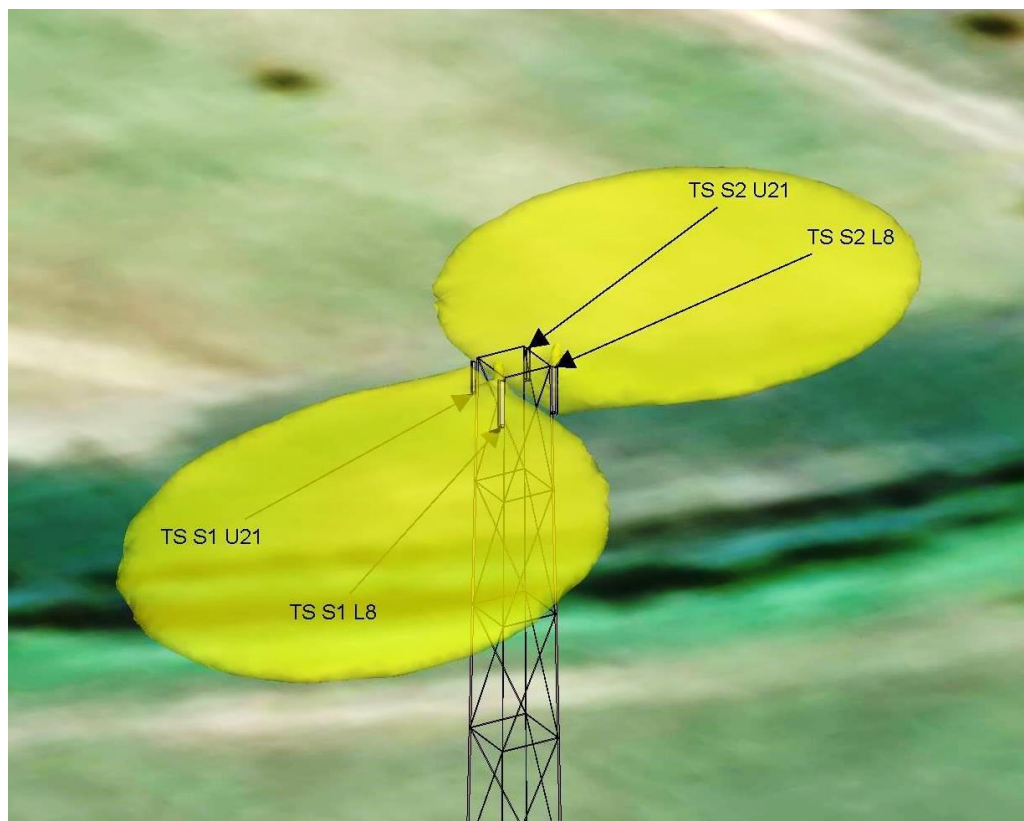
Slika 6.7 Prikaz polja koje stvaraju antene pri maksimalnom opterećenju, pogled iz perspektive
