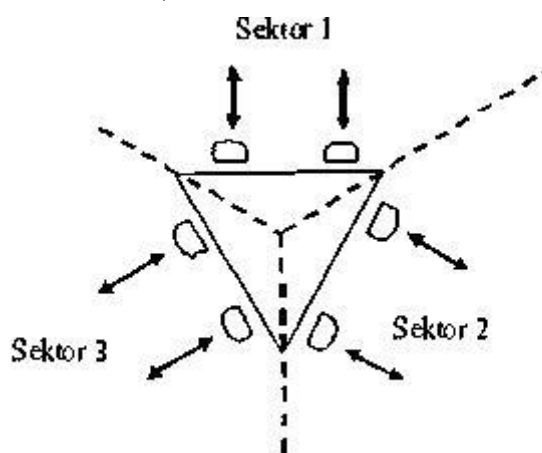
Slika 3.3 Trosektorski sistem GSM
