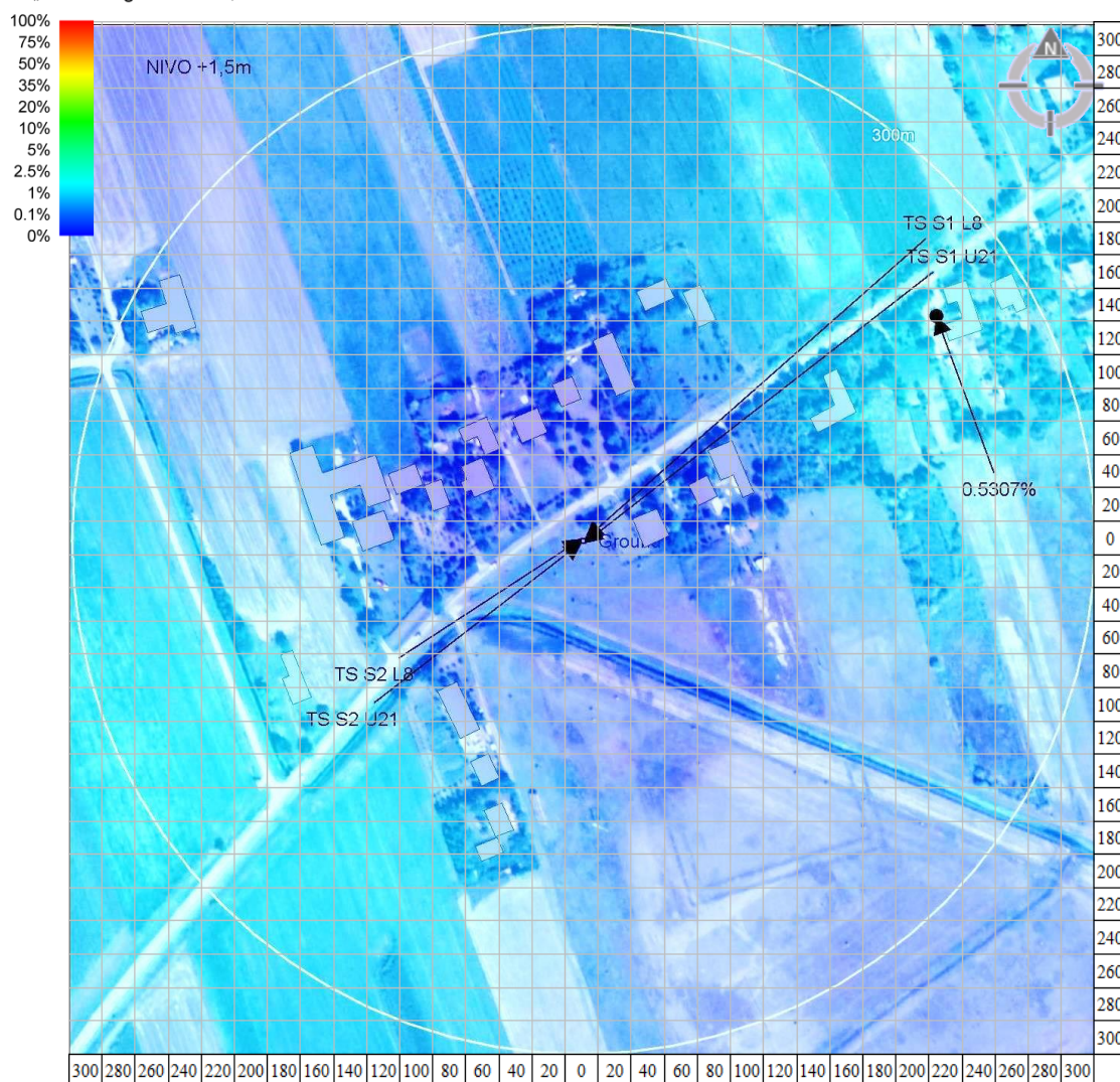
Slika 6.10. Jačina električnog polja radio-sistema UMTS2100 i LTE800 bazne stanice „SOU73, SOO73 SOMBOR OBZIR” operatora „Telekom Srbija” na nivou 1,5 m
