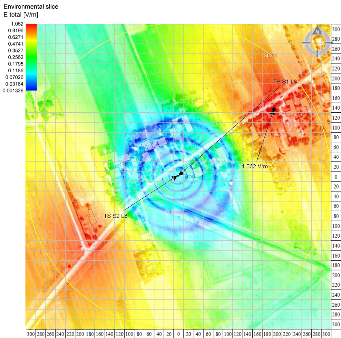
Slika 6.9. Jačina električnog polja radio-sistema LTE800 bazne stanice „SOU73, SOO73 SOMBOR OBZIR” operatora „Telekom Srbija” na nivou 1,5 m
