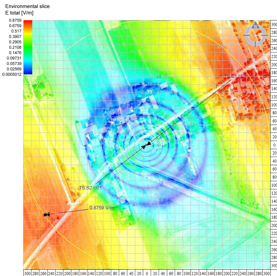
Slika 6.8. Jačina električnog polja radio-sistema UMTS2100 bazne stanice „SOU73, SOO73 SOMBOR OBZIR” operatora „Telekom Srbija” na nivou 1,5 m
