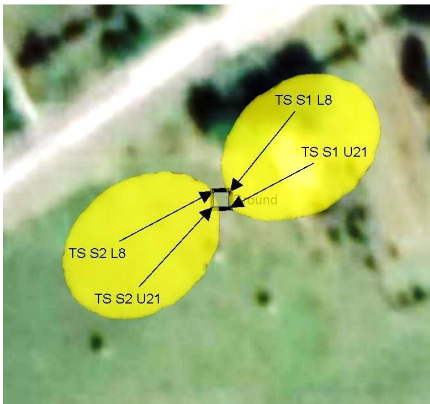
Slika 6.4 Prikaz polja koje stvaraju antene pri maksimalnom opterećenju, pogled iz perspektive
