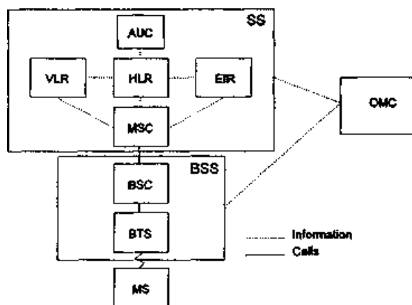
Slika 3.2 Blok dijagram GSM mobilne telefonske mreže
