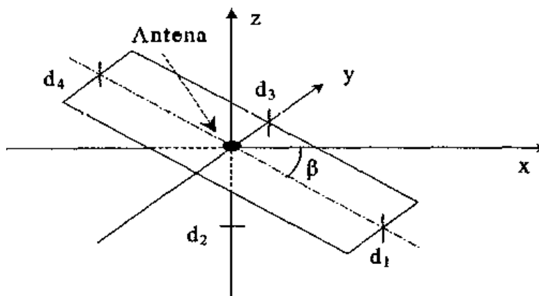
Slika 6.2 Rastojanja od antene, za koja se definiše maksimalna vrednost intenziteta vektora jačine električnog polja E_{max}
