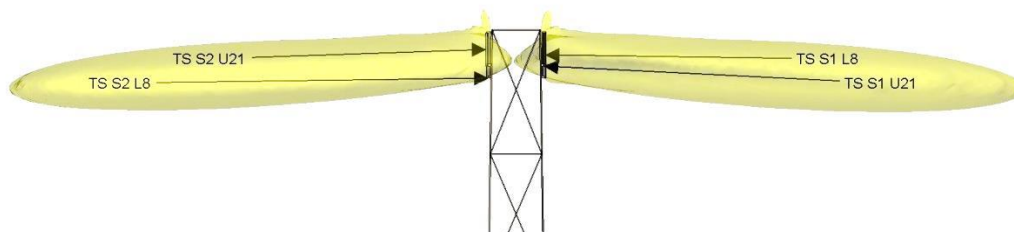
Slika 6.6 Kontrolisana zona, horizontalan pogled na antene iz pravca istoka
