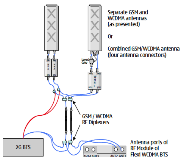
Slika 3.4 Princip kombinacije GSM i WCDMA baznih stanica
