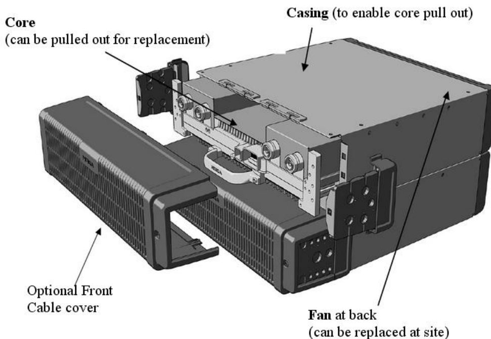
Slika 3.6 Prikaz dvostrukog radio modula za realizaciju UMTS meže
