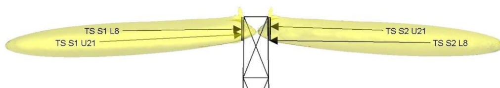
Slika 6.5 Kontrolisana zona, horizontalan pogled na antene iz pravca zapada
