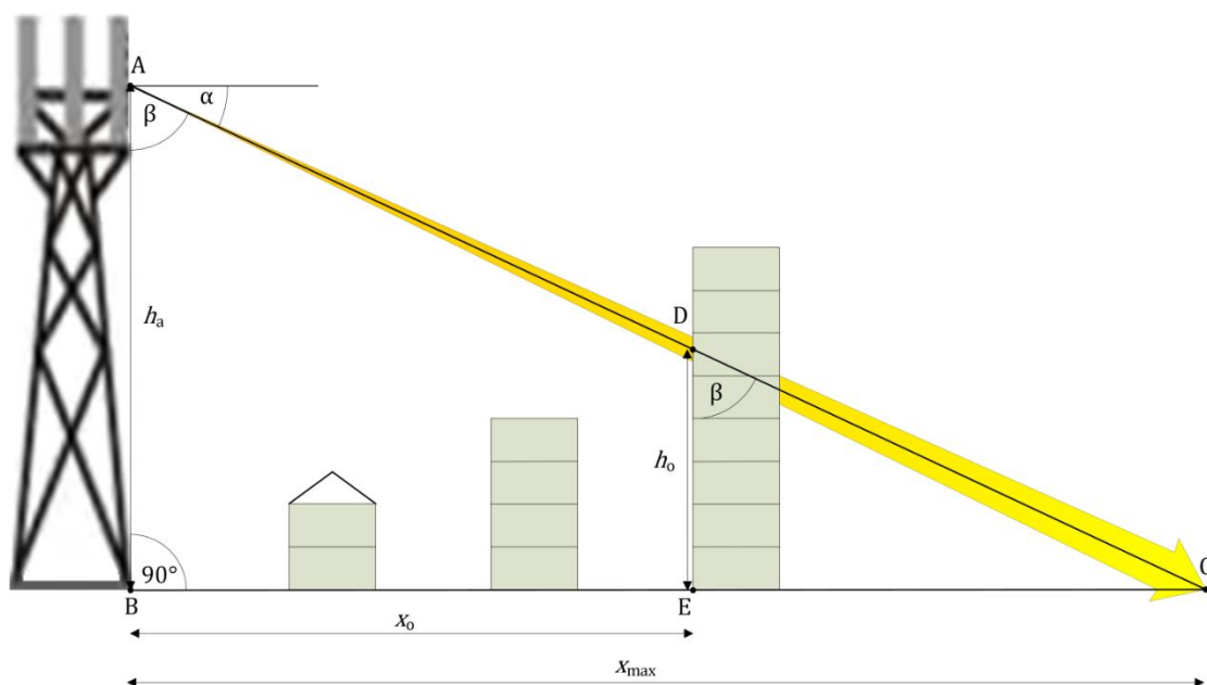
Slika 6.1B Određivanje najizloženijeg sprata objekta u zoni povećane osetljivosti
