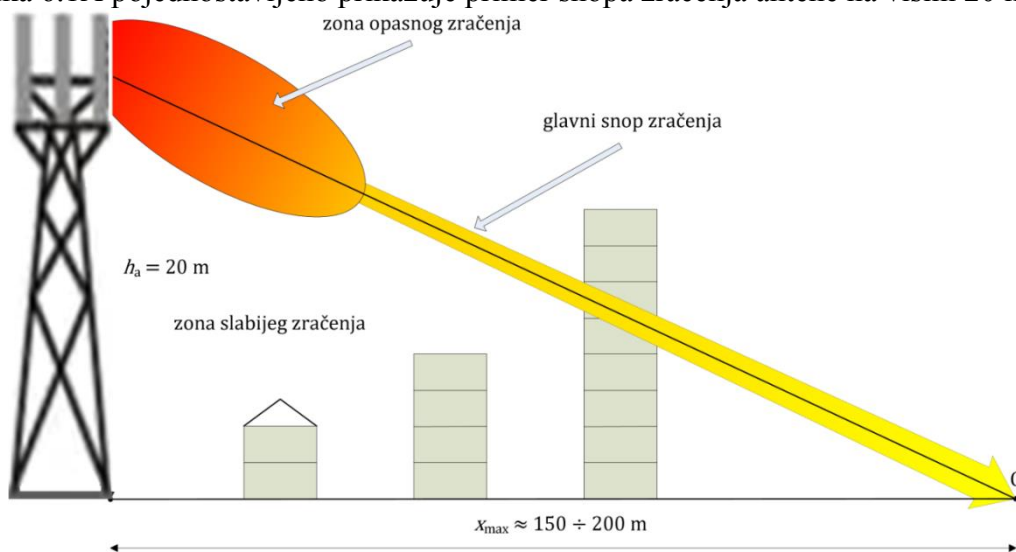
Slika 6.1A Primer snopa zračenja antene na visini 20 m
