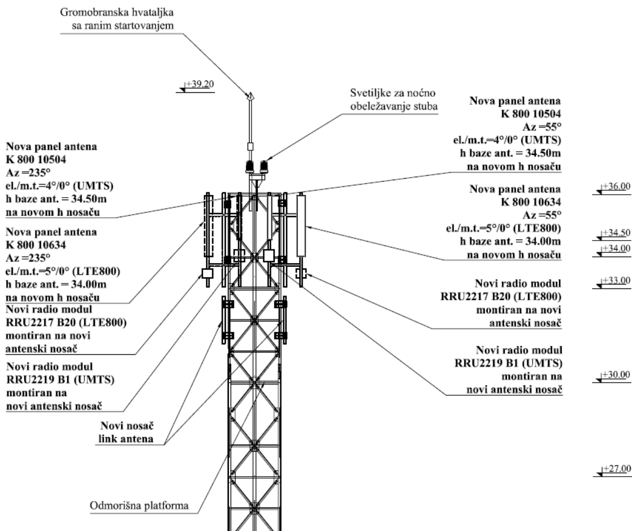
Slika 4.2 Slika antenskog stuba sa antenama
