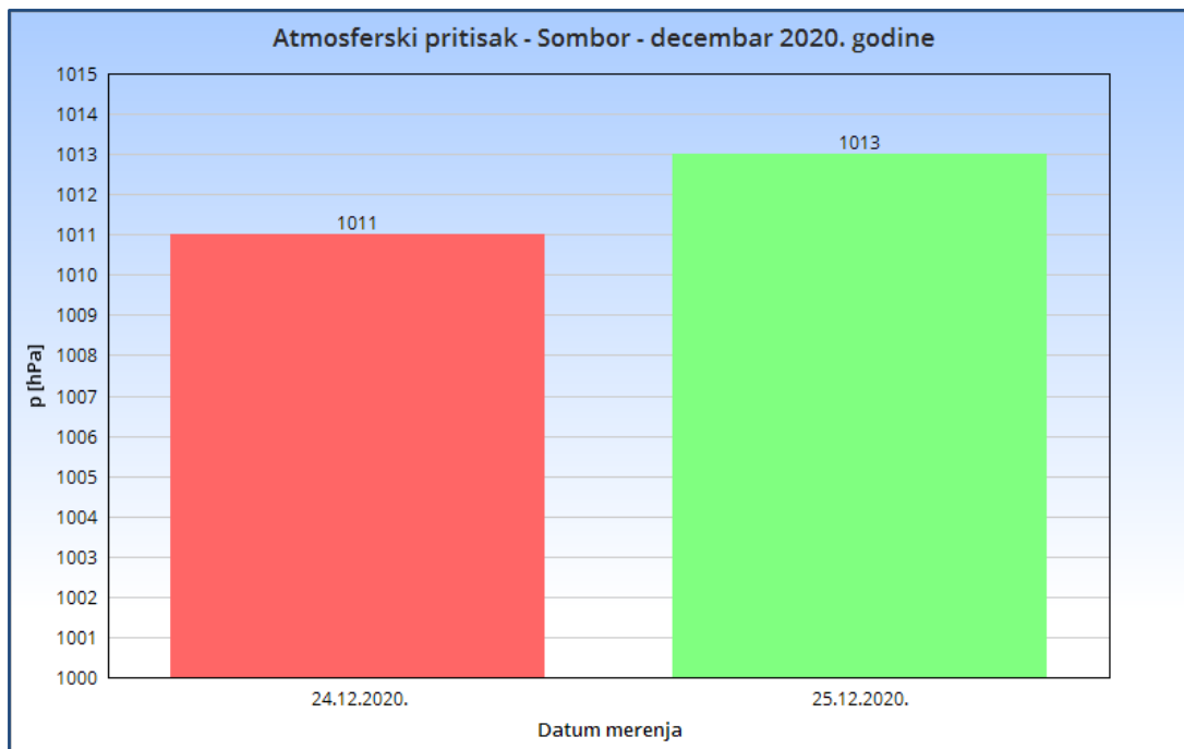
Slika 2.3. Atmosferski pritisak - Sombor decembar 2020. godine
