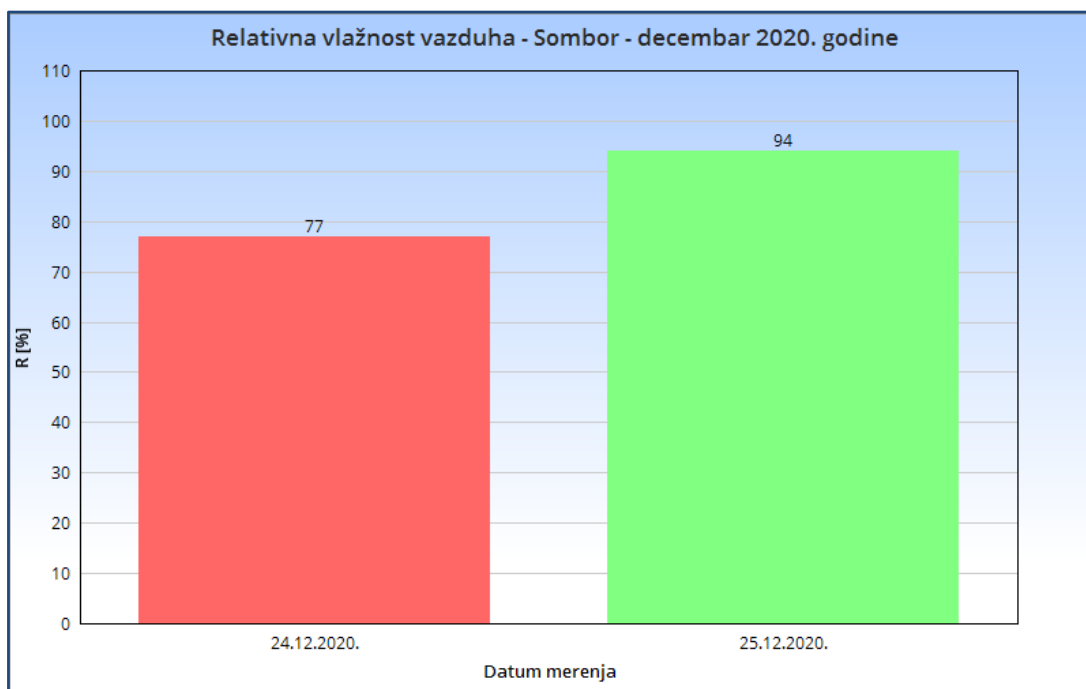
Slika 2.2. Relativna vlažnost vazduha - Sombor decembar 2020. godine
