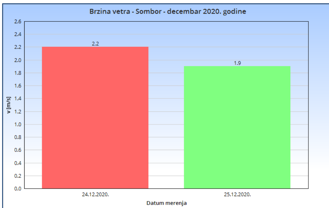
Slika 2.4. Brzina vetra - Sombor decembar 2020. godine
