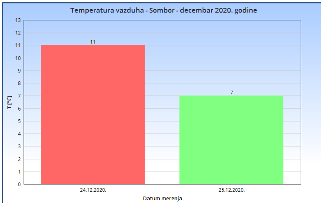
Slika 2.1. Temperatura vazduha - Sombor decembar 2020. godine
