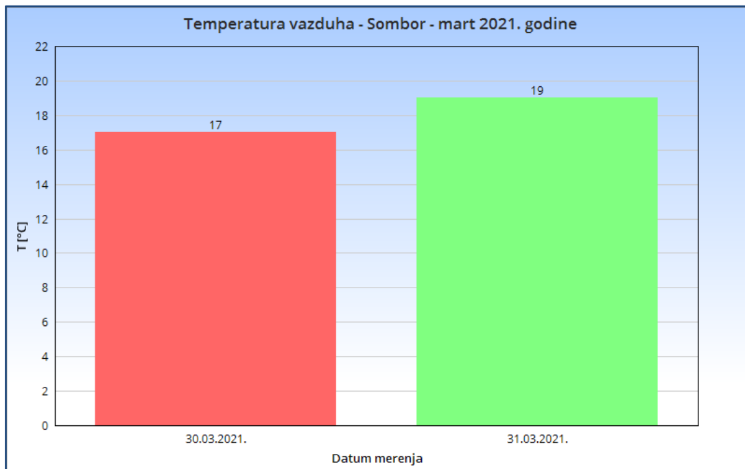
Slika 2.1. Temperatura vazduha - Sombor mart 2021. godine
