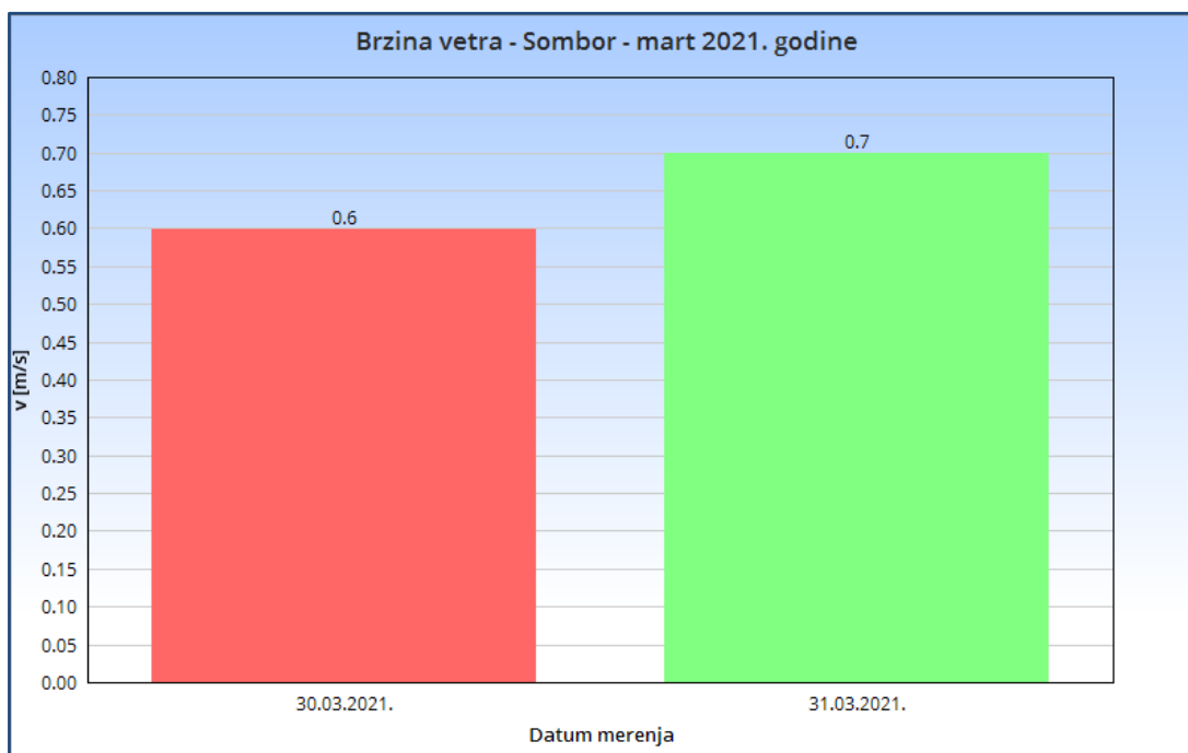
Slika 2.4. Brzina vetra - Sombor mart 2021. godine
