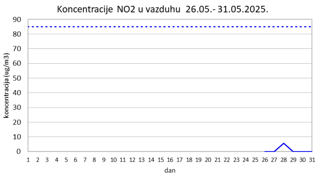
Grafik 3 : Koncentracija NO 2 u periodu 26.05.- 31.05.2025. na lokaciji Dvorište Zavoda za javno zdravlje Sombor
